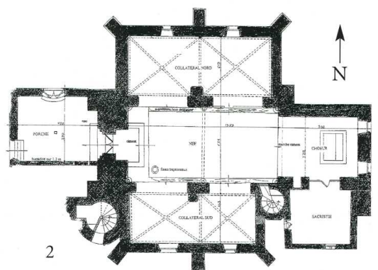
Arx (Landes) Église Saint-Martin 1. Façade méridionale 2. Plan (Architecture Patrimoine, 1998)
