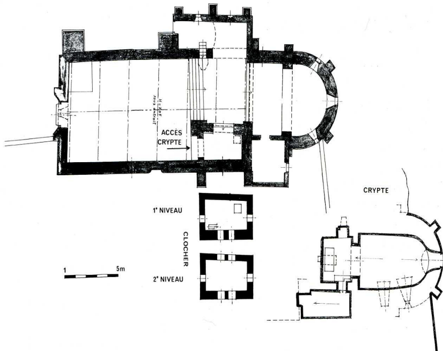
Avril-sur-Loire (Nièvre). Plan de l'église Saint-Pierre et de sa crypte.
