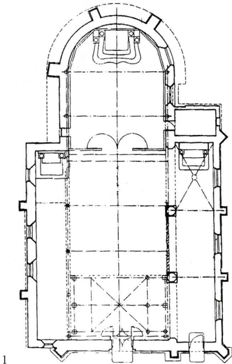
Beauche (Eure-et-Loir) Église Saint-Martin 1. Plan (J.L. Latour et R. Martin, arch.) 2. Façade sud
