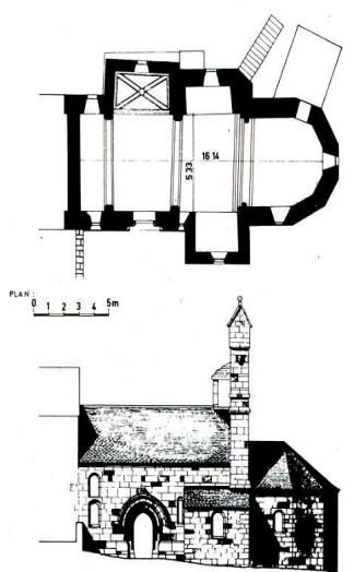
Blavignac (Lozère). Église Saint-Julien, plan et élévation de la façade sud.
