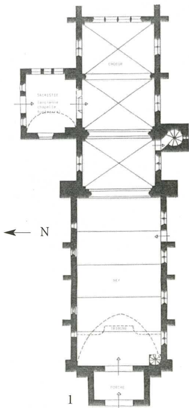
Bouquetot (Eure) Église Saint-Philbert 1. Plan 2. Élévation sud de l'église et porche
