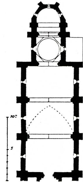
Braize (Allier), église Saint-Antoine. Plan n.s.n.d.
