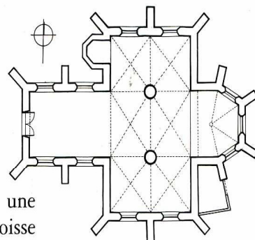
Bucey-en-Othe (Aube). Plan de l'église Saint-Jacques.
