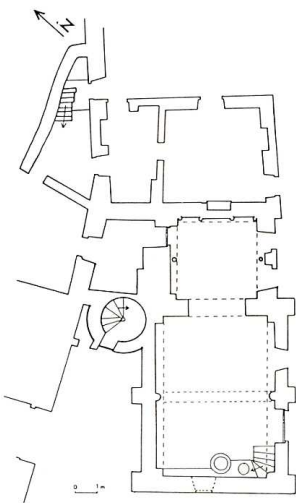
Champeix (Puy-de-Dôme). Chapelle Saint-Jean, plan.
