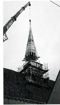
Charray (Eure-et-Loir), église Saint-Marcel, mise en place de la charpente du clocher.
