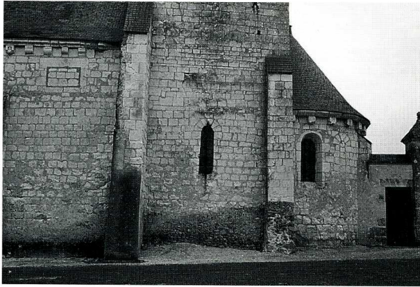
Chartrené (Maine-et-Loire), église Saint-Maurice. 1. Façade sud et chevet. 2. Plan, éch. 0,01, 1960.
