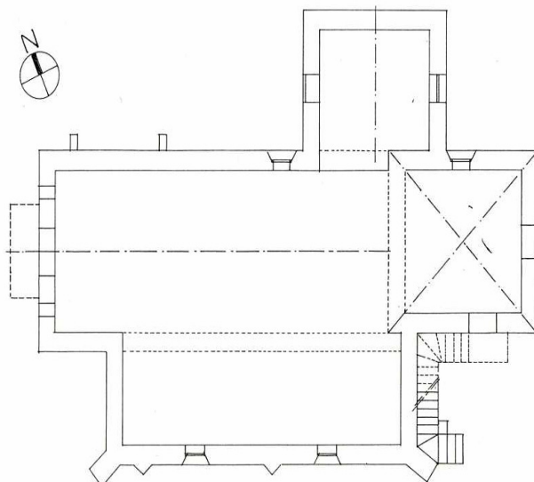
Chavannes (Drôme), église Saint-Priest, plan d'ensemble de l'église, par Evelyne et Charles Colomb, arch., éch. 0,01 (juillet 1993).
