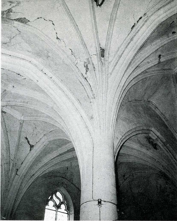
Chervey (Aube).
