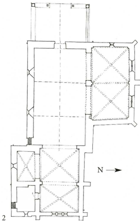
Crans (Ain) Église Notre-Dame 1. Chevet 2. Plan (Ph. Allart, arch.) 1997
