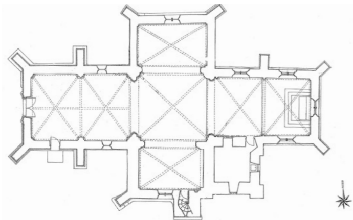
2. Plan (Antoine Leriche, arch. du patrimoine)
