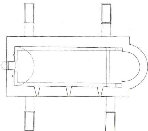
Fontvieille (Bouches-du-Rhône), chapelle Saint-Jean. 1. Plan, éch. 0,01. 2. Élévation de la façade ouest. 3. Élévation de la façade sud. Agence des Bâtiments de France, 1994.
