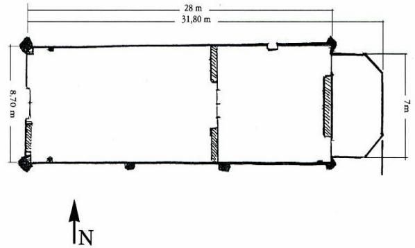
Grosley-sur-Risle (Eure) Eglise Saint-Léger. Schéma.
