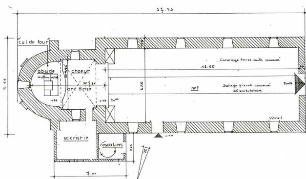
Huilly-sur-Seille (Saône-et-Loire), église Saint-Georges, plan de l'église établi par G. Golion, arch., éch. 0,01 (1993).
