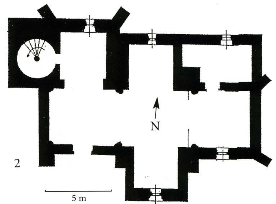
Lacapelle-Ségalar (Tarn) Église Sainte-Cécile 2. Relevé (Th. Casel, arch., 2001)
