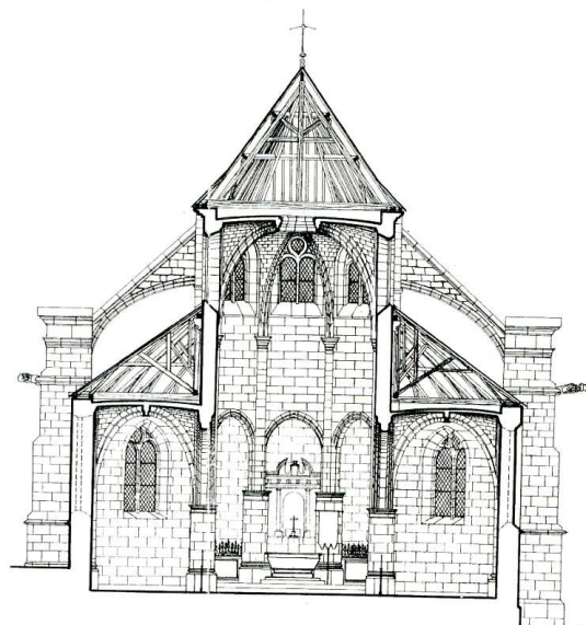
Lavau (Yonne), église Saint-Germain. 1. Coupe sur le chœur, éch. 0,01, H. Cazelles, arch., 1993. 2. Chœur.
