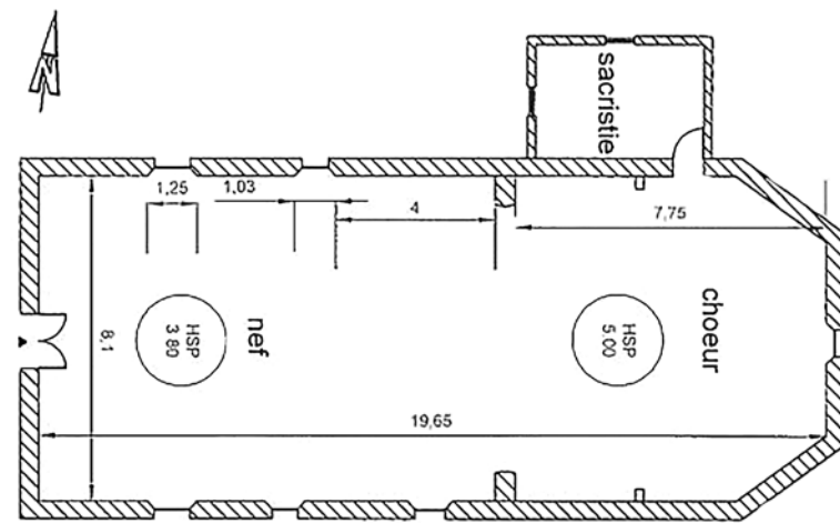
2. Schéma (éch.1/100 e )
