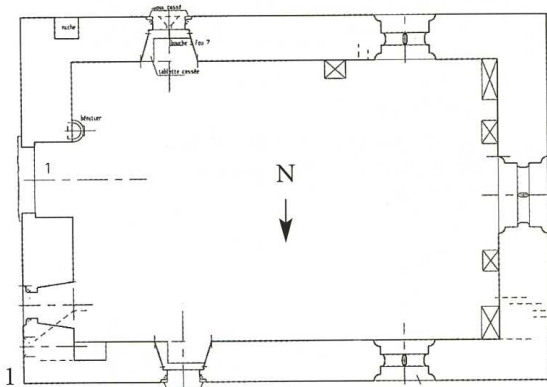
Locmaria-Plouzané (Finistère) Chapelle Saint-Claude 1. Plan (Fr. Cadiou, arch.) 2. Façade sud (cl. T. Daniel)
