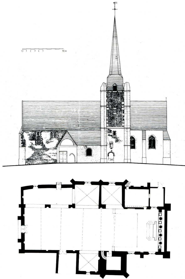
Marçon (Sarthe). Église Notre-Dame, façade sud et plan.
