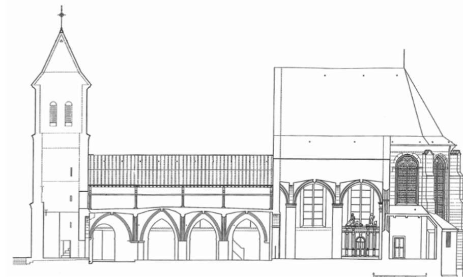
3. Coupe longitudinale
