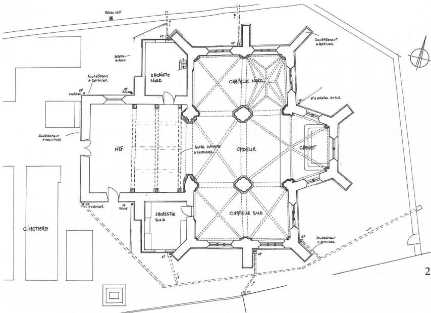
2. Plan (A. Leriche, arch.)
