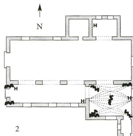
Requeil (Sarthe) Église Saint-Pierre 1. Façade sud 2. Plan avec indication des fissures (Adès) 1993
