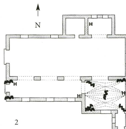
Requeil (Sarthe) Église Saint-Pierre 1. Façade sud 2. Plan avec indication des fissures (Adès) 1993
