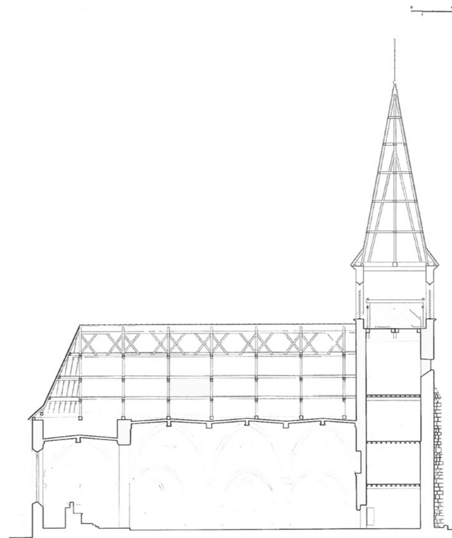
4. Coupe longitudinale ouest-est (Patrice Salès, arch. du patrimoine)
