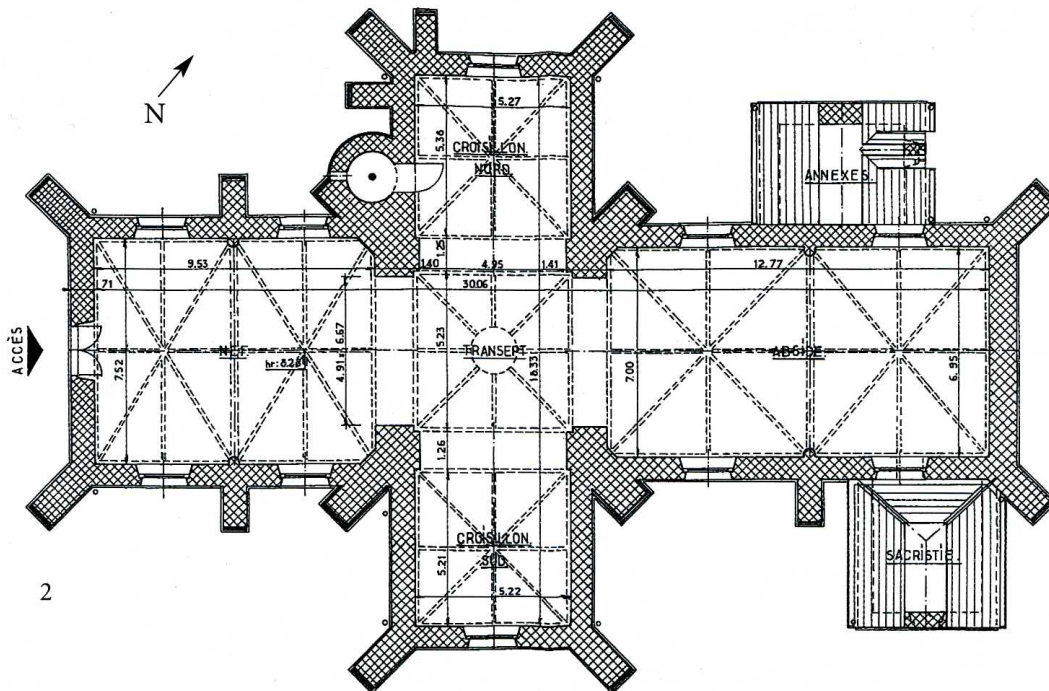
Saint-Léger-Vauban (Yonne) Église Saint-Léger 2. Plan (Y. Botte)
