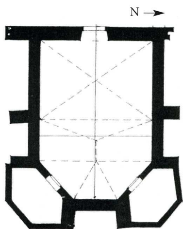
Seringes-et-Nesles (Aisne) Chapelle Saint-Nicolas de Nesles 1. Vue générale du chevet (cl. J.-Cl. Druésne) 2. Plan (A. et O. Gigot, arch., 1999)
