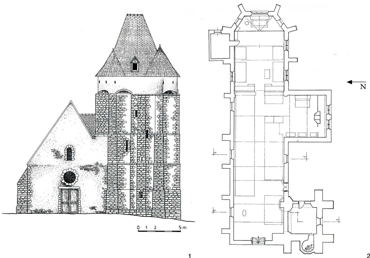
Soucy (Yonne). Église Saint-Étienne. 1- Élévation ouest, éch. 0,005 (Th. Algrin et H. Cazelles, arch. 1999) . 2- Plan, éch. 0,005 (Th. Algrin et H. Cazelles, arch. 1999).
