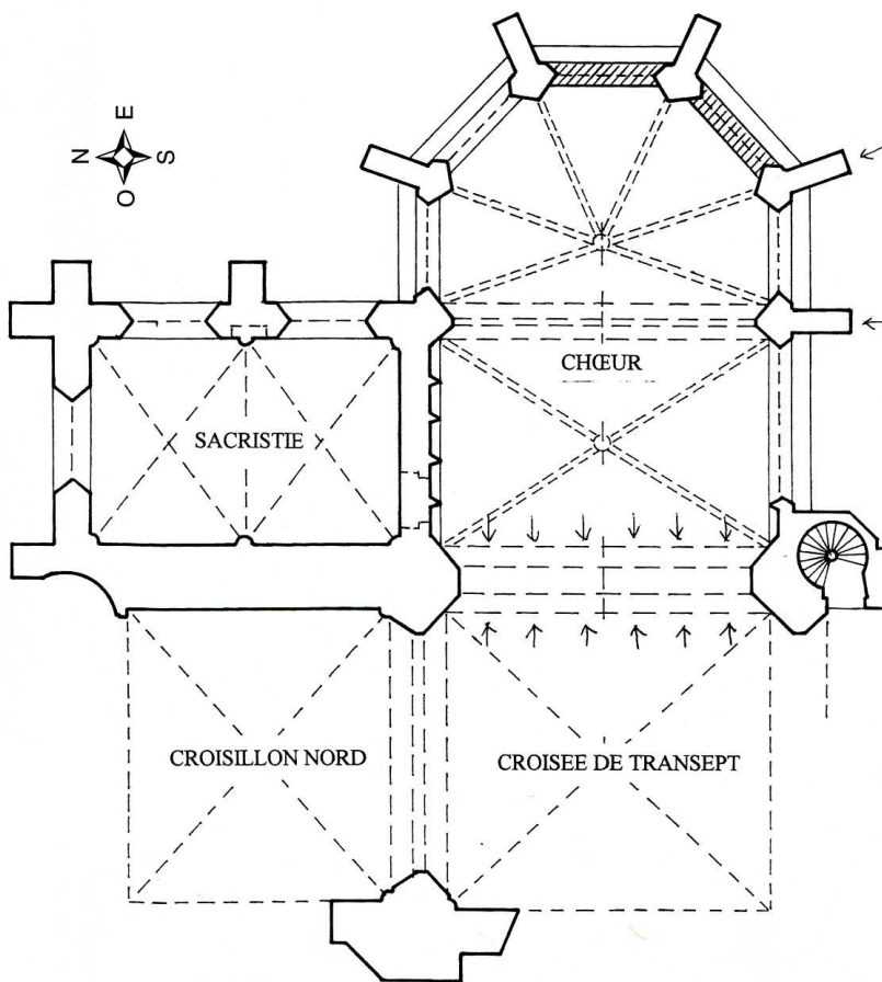
Tilly (Eure) Église Notre-Dame de Saulseuse Plan J.-P. Soyez
