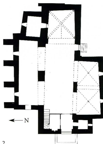
Valernes (Alpes-de-Haute-Provence) Église Sainte-Marie-Madeleine 1. Vue du sud-ouest (cl. J. Huguet) 2. Plan (SDAP)
