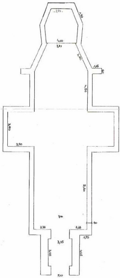
Vaudéville (Vosges), église Saint-Quirin. Plan schématique, éch. 0,01, n.s.n.d.
