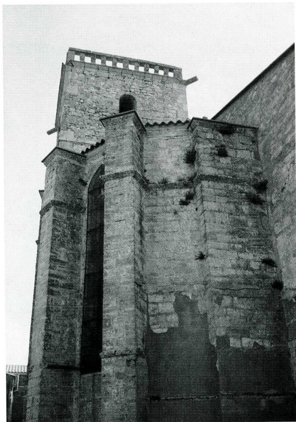
Vendres (Hérault). Église Saint-Étienne, chevet et plan. (Y. Poussines, architecte, 1990).
