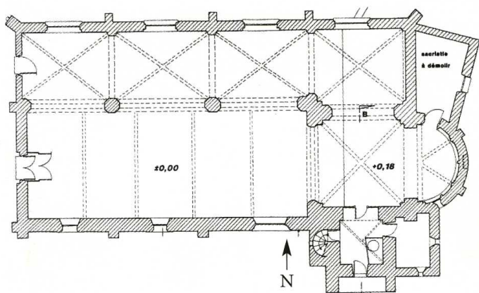
Viabon (Eure-et-Loir) Église Saint-Martin 2. Plan (J.-P. Esnault, arch. 2001) 3. Charpente de l'abside
